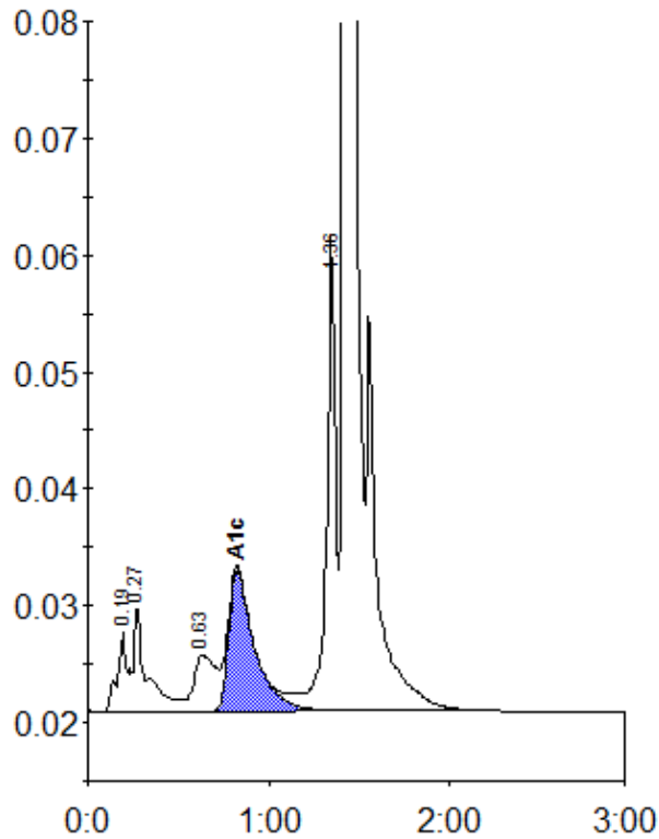
Peak table - ID: DPLTA00254209
