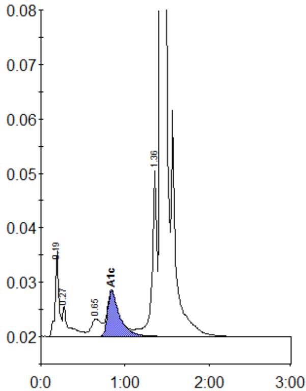
Peak table - ID: 10653945
