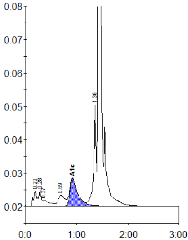
Peak table - ID: 10678355
