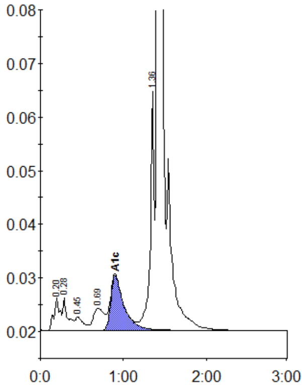
Peak table - ID: 10637601
