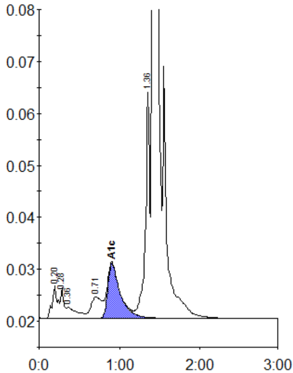
Peak table - ID: 10546229
