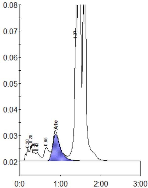
Peak table - ID: 10616279
