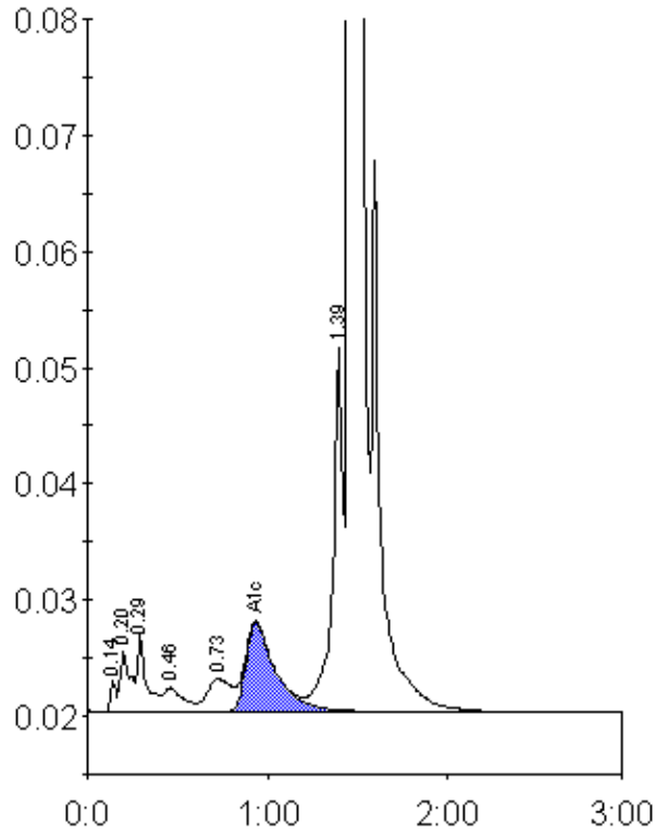
Peak table - ID: 10596264
