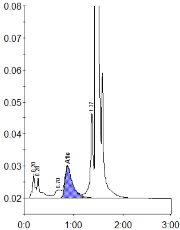
Peak table - ID: 10337172
