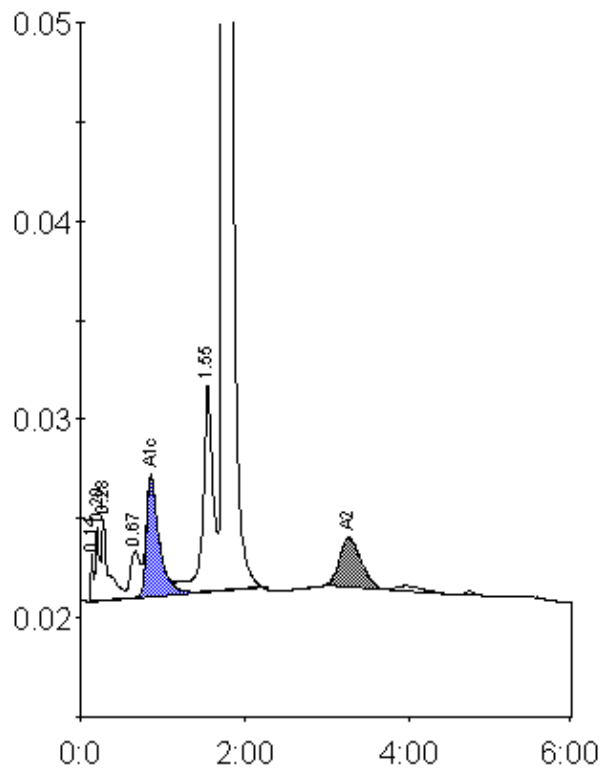
Peak table - ID: 10360587
