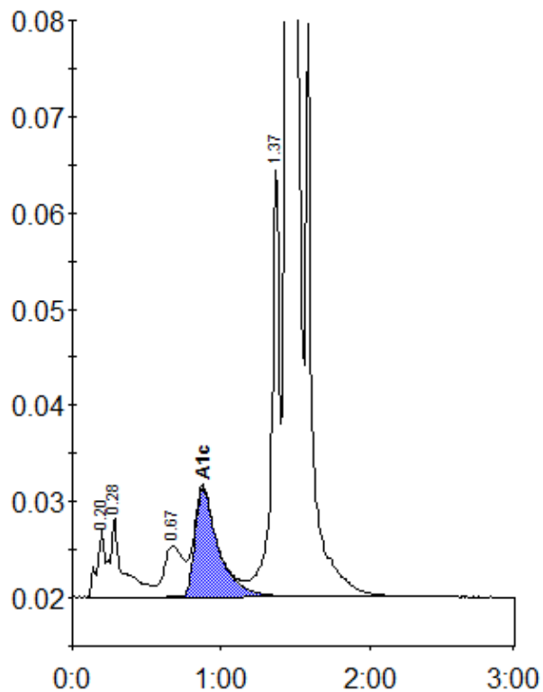
Peak table - ID: 10341679
