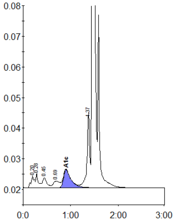
Peak table - ID: 10400048
