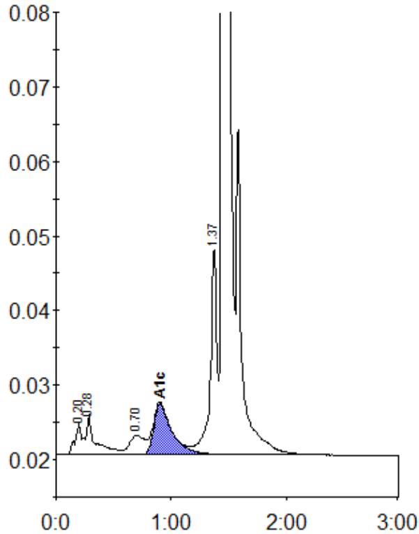
Peak table - ID: 10363170
