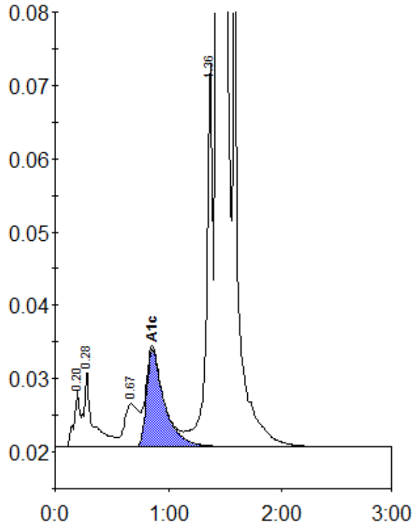
Peak table - ID: 10292315
