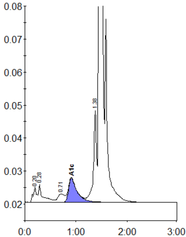
Peak table - ID: 10251448
