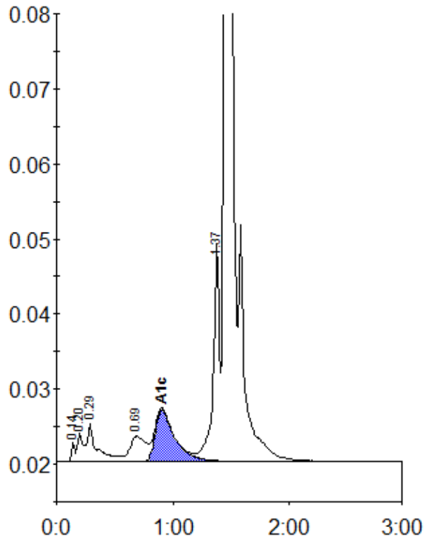
Peak table - ID: 10329187
