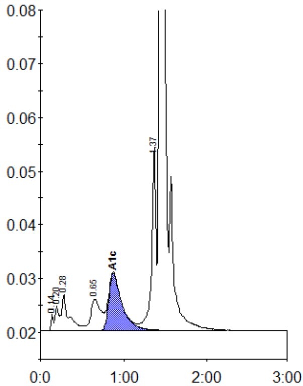
Peak table - ID: 10299294
