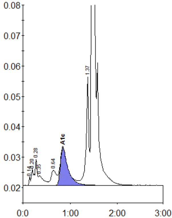
Peak table - ID: 10197871
