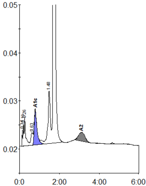
Peak table - ID: 10162253
