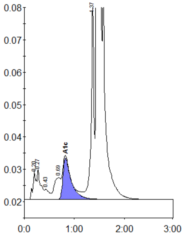
Peak table - ID: 10136748
