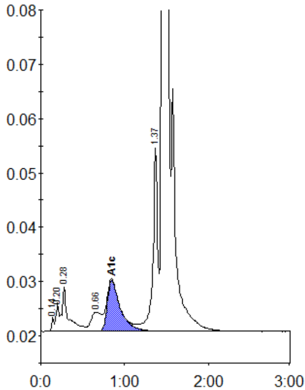
Peak table - ID: 10162515
