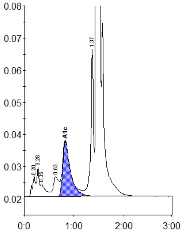
Peak table - ID: 10166714
