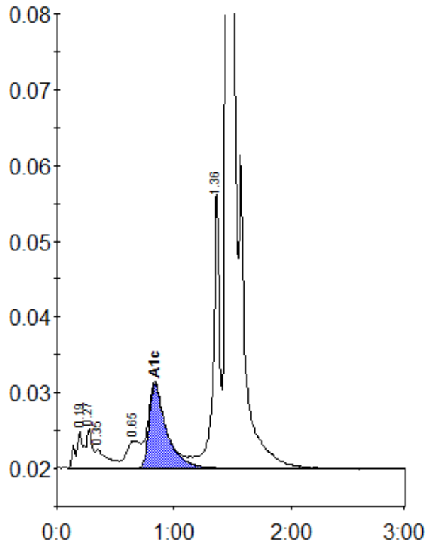
Peak table - ID: 10176718
