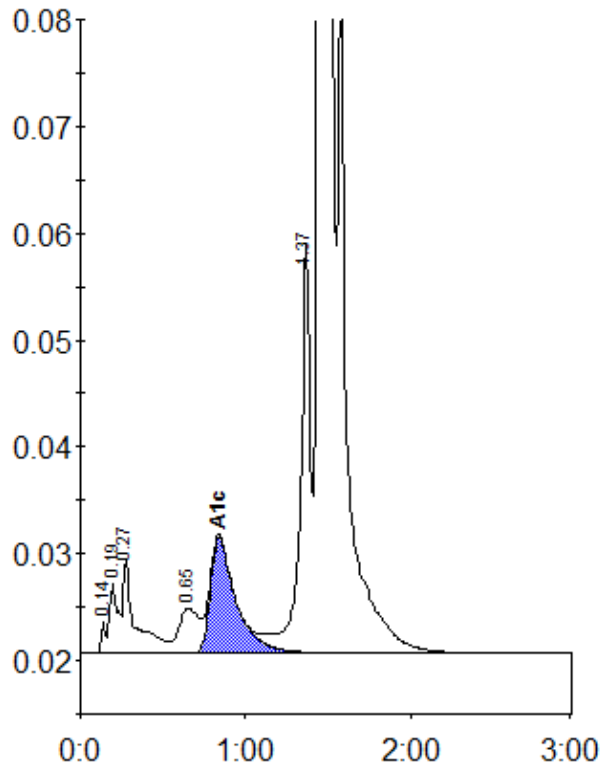
Peak table - ID: 10158993
