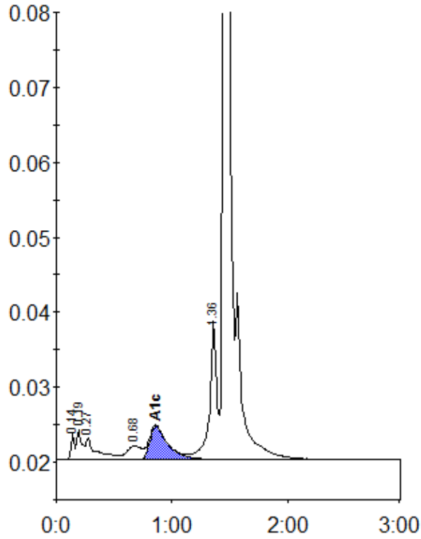
Peak table - ID: 10159279
