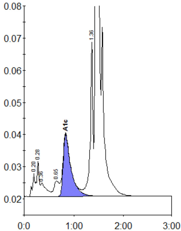
Peak table - ID: 10142479
