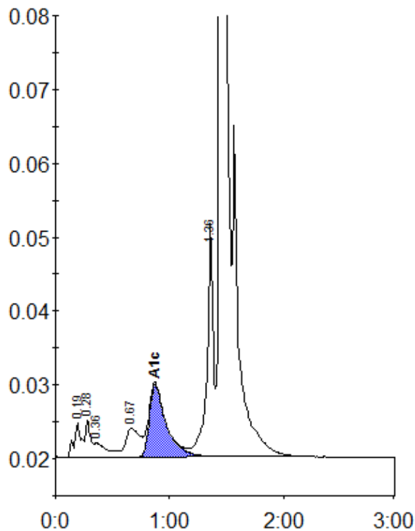
Peak table - ID: 0086659
