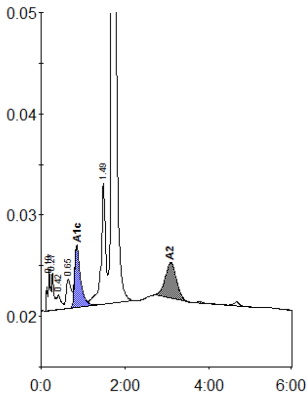
Peak table - ID: 10109676
