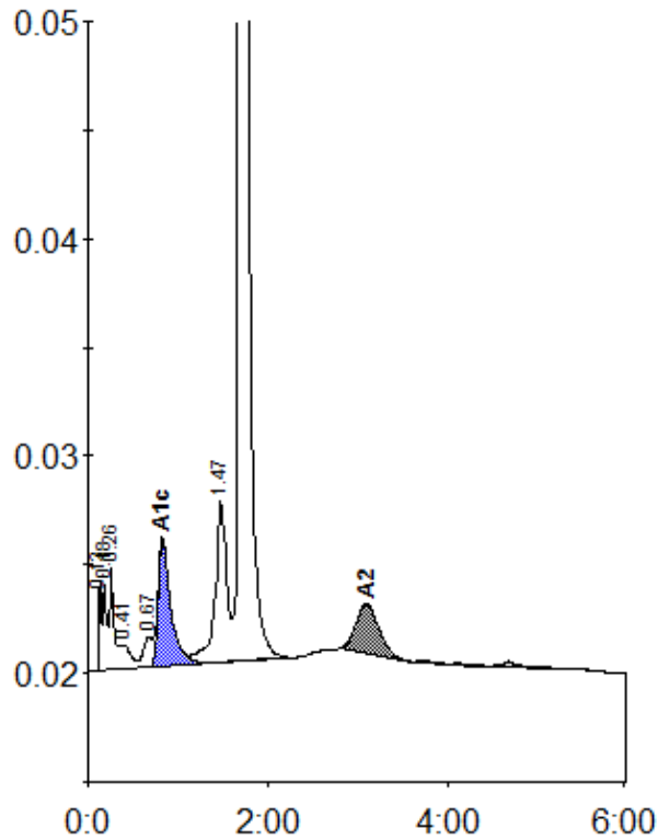
Peak table - ID: 10028346
