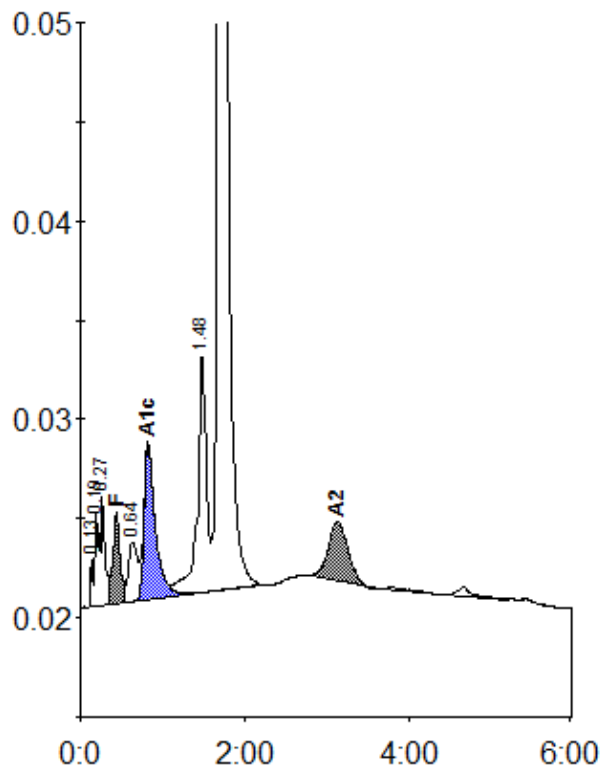
Peak table - ID: 10005572
