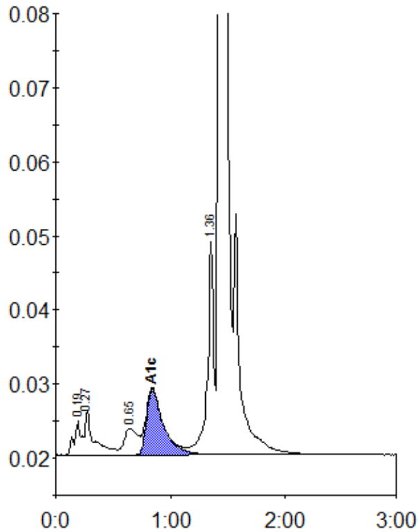
Peak table - ID: 10005170
