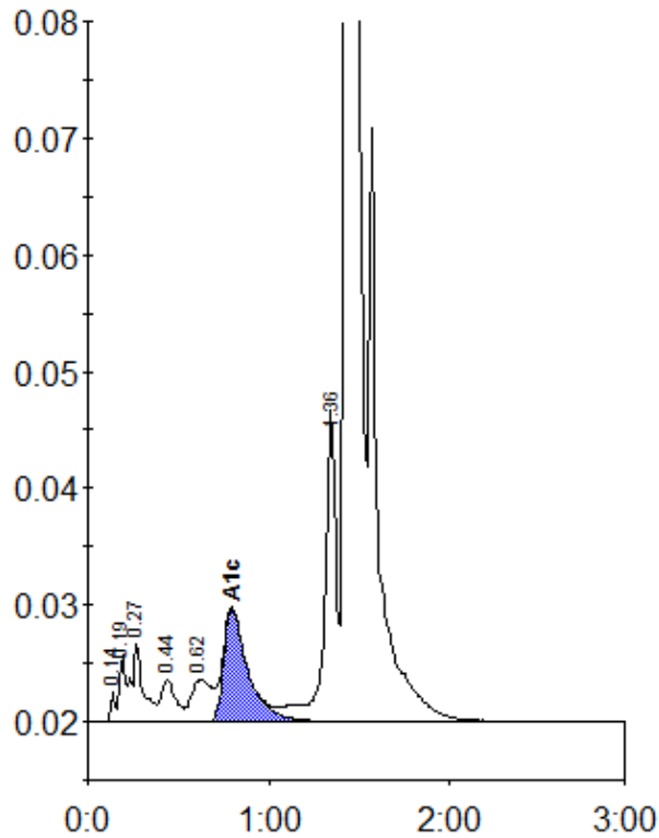
Peak table - ID: 01040041
