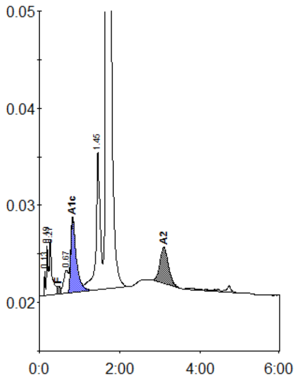
Peak table - ID: 01300075
